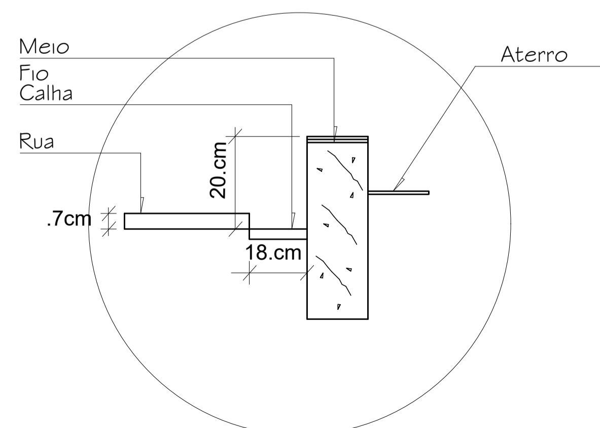
02 DETALHAMENTO SARGETA SEM ESCALA
